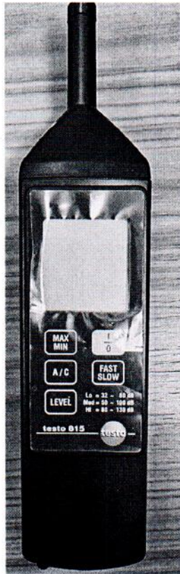
Рисунок 1.1 – Фотография общего вида измерителя уровня звука testo 815 № 30831033/102
