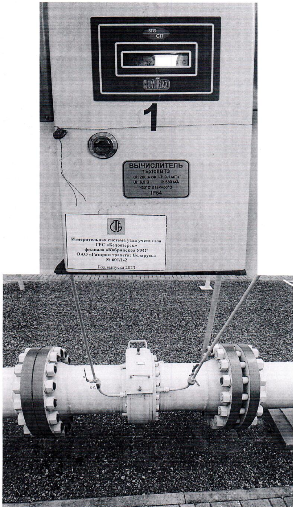
Рисунок 1.1 – Фотографии общего вида ИС УУГ
