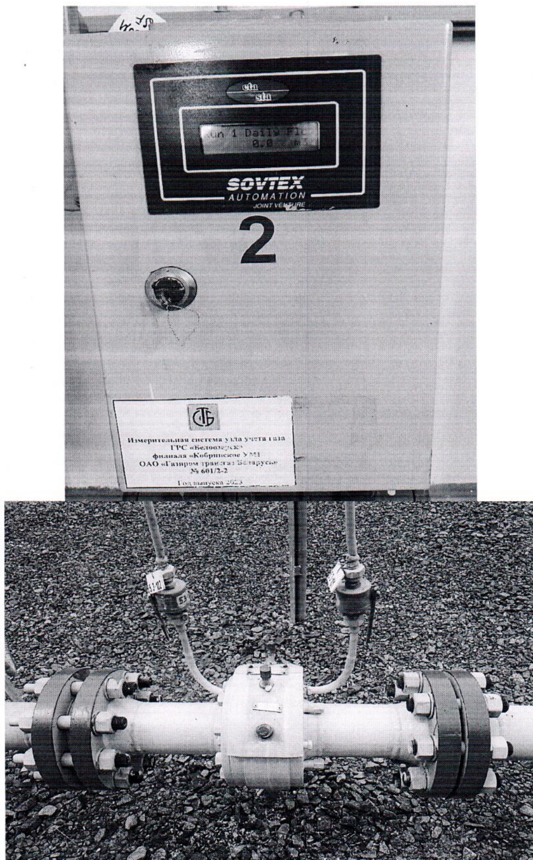
Рисунок 1.1 – Фотографии общего вида ИС УУГ
