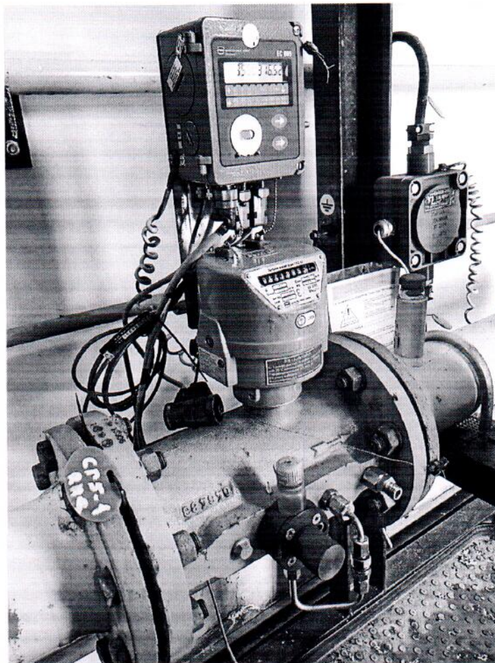
Рисунок 1.1 – Фотография общего вида ИС УУГ
