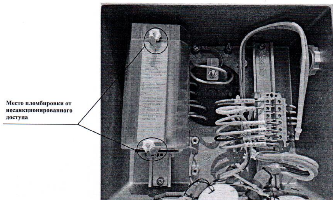
Рисунок 3 - Схема пломбировки от несанкционированного доступа
