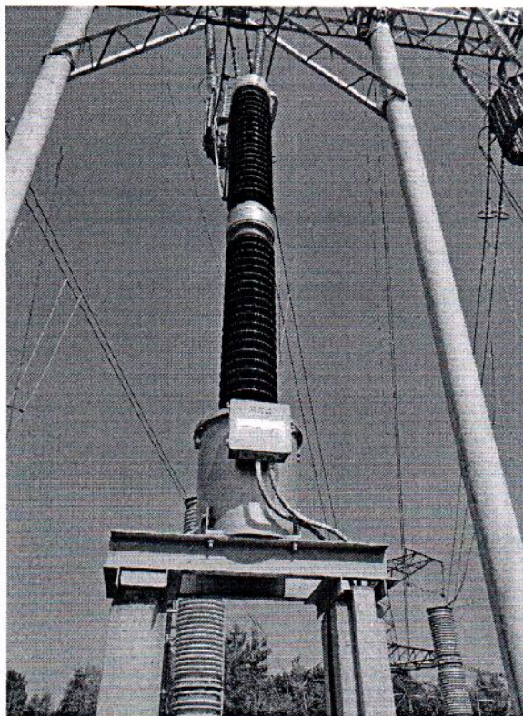
Рисунок 1 - Фотография общего вида трансформатора напряжения емкостного типа СРВ 362 № 1HSE 8804603
