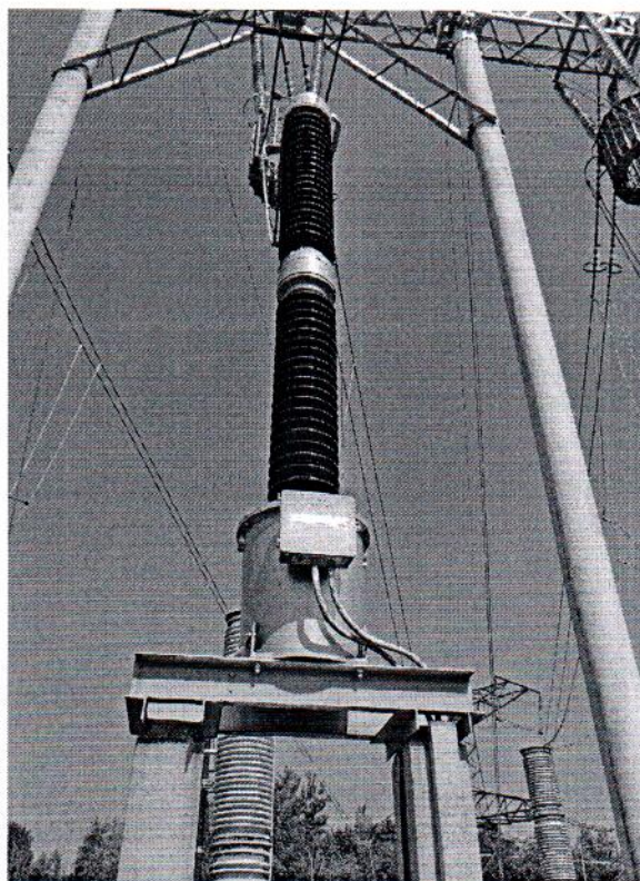
Рисунок 1 - Фотография общего вида трансформатора напряжения емкостного типа СВН 362 № 1HSE 8804602
