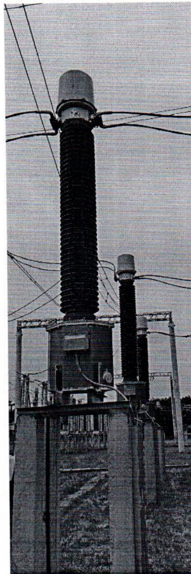
Рисунок 1 - Фотография общего вида трансформатора тока типа IMB 362 №1HSE 8804599
