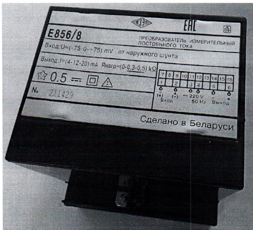
Рисунок 1 – Общий вид и маркировка ИП E856/8 для нужд народного хозяйства
