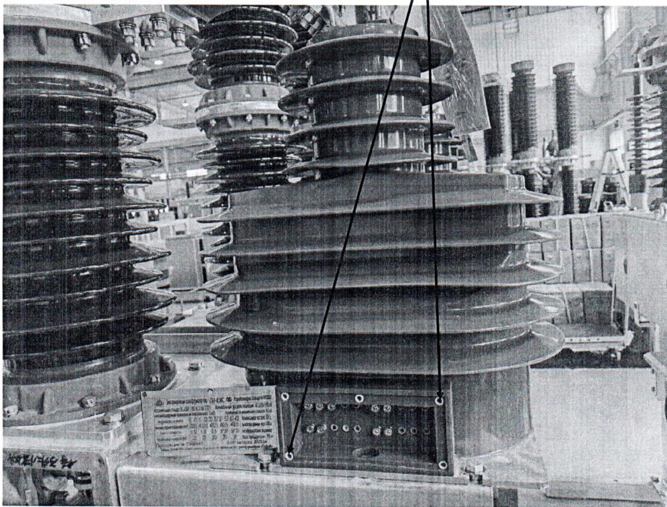
Рисунок 3 – Фотография пломбировки от несанкционированного доступа трансформатора тока LZZBJ9-40.5WC № 2306997
