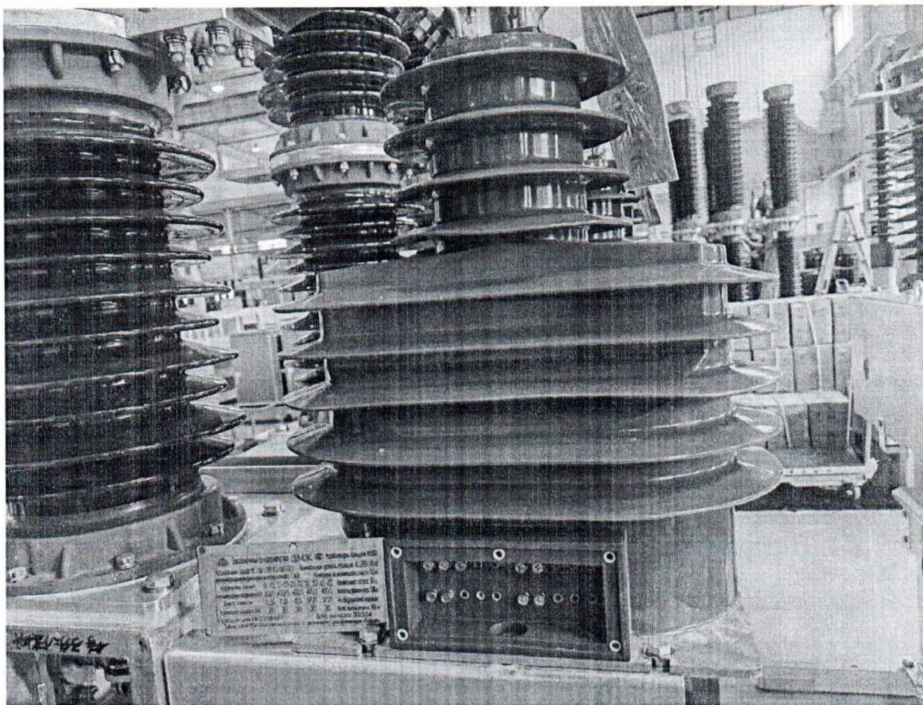
Рисунок 1 – Фотография общего вида трансформатора тока LZZBJ9-40.5WC № 2306997
