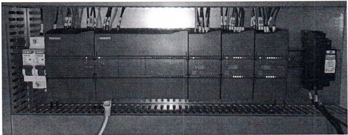
Фотография 7 – Контроллер программируемый SIMATIC S7-1200
