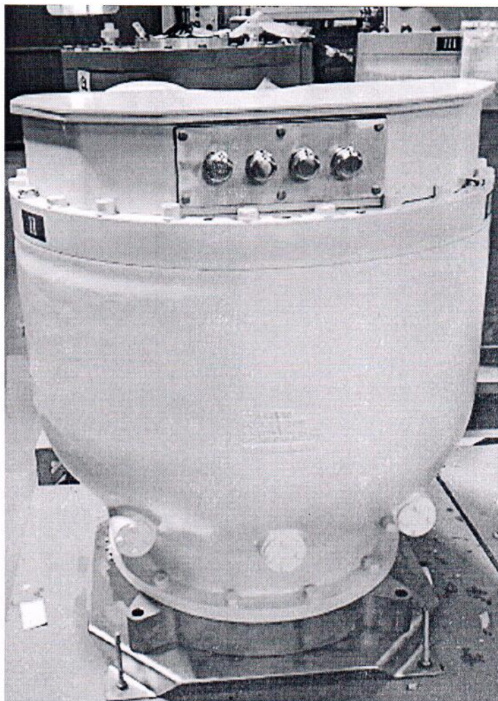
Рисунок 1.1 – Фотографии общего вида трансформатора напряжения SU145/S92 № 1VT564
