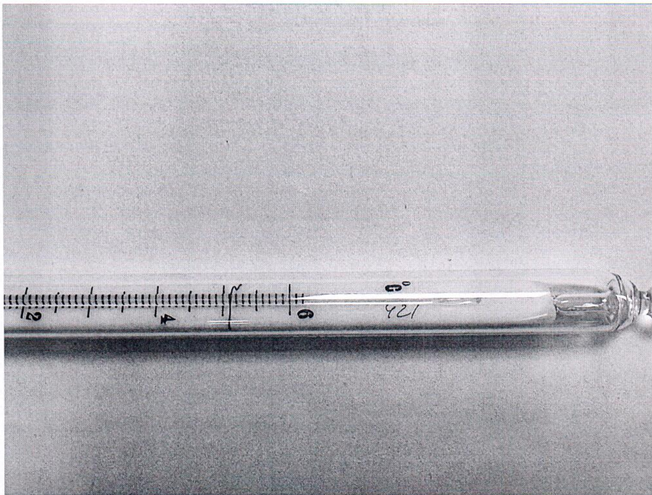
Рисунок 1.2 – Фотография маркировки термометра стеклянного ртутного СП-74 № 5 заводской № 421
