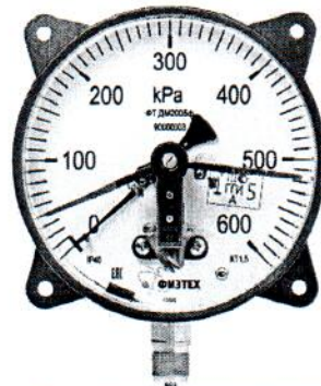
Рисунок 4 – Приборы электроконтактные (сигнализирующие)
