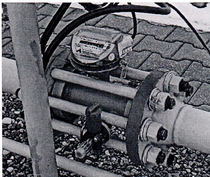
Рисунок 1.1 – Фотографии общего вида ИС УУГ
