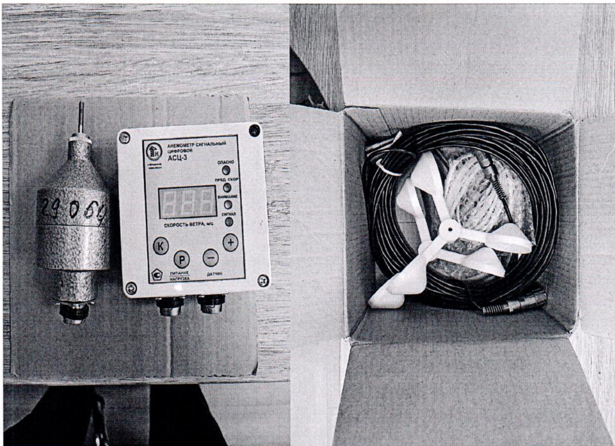
Рисунок 1.1 – Фотография общего вида анемометра сигнального цифрового АСЦ-3 № 29064
