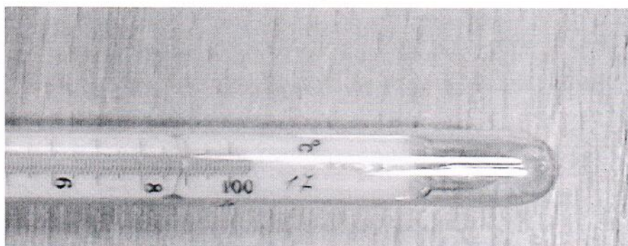
Рисунок 1.2 – Фотография маркировки термометра лабораторного стеклянного с взаимозаменяемыми конусами № 3, заводской № 17
