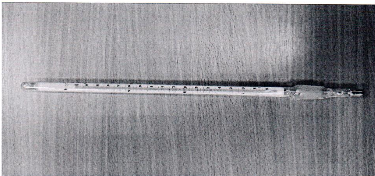
Рисунок 1.1 – Фотография общего вида термометра лабораторного стеклянного с взаимозаменяемыми конусами № 3, заводской № 8
