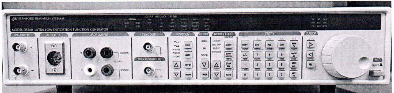
Рисунок 1.1 – Фотография общего вида генератора сигналов DS360 № 61752
