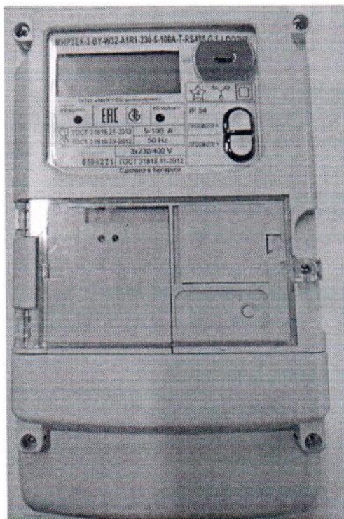
Рисунок 1.3 – Фотография общего вида счётчика «МИРТЕК-3-ВУ» в типе корпуса «W32», «W33», «W37», «W38»
