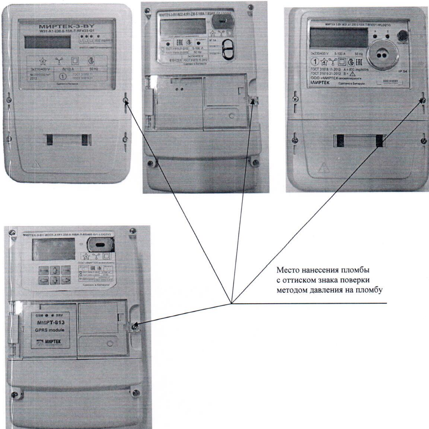
Рисунок 3.1 – Схема пломбировки счетчика от несанкционированного доступа
