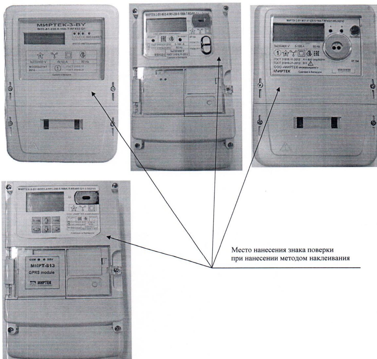
Рисунок 2.1 – Схема (рисунок) с указанием места для нанесения знаков поверки на счётчики
