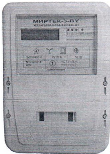
Рисунок 1.1 – Фотография общего вида счётчика «МИРТЕК-3-ВУ» в типе корпуса «W31», «W34», «W35», «W36»
