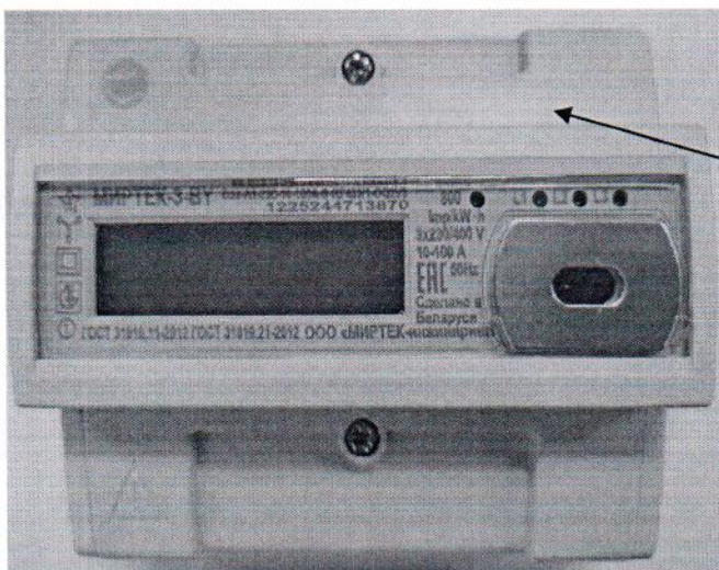
Рисунок 2.2 – Схема (рисунок) с указанием места для нанесения знаков поверки на счётчики
