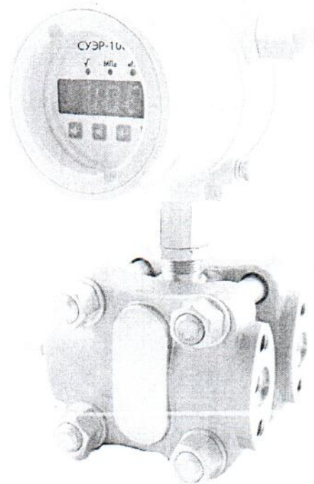
Рисунок 6 - Общий вид фланцевых датчиков давления СУЭP-100-ДИ, СУЭP-100-ДА, СУЭP-100-ДВ, СУЭP-100-ДИВ, СУЭP-100-ДД.
