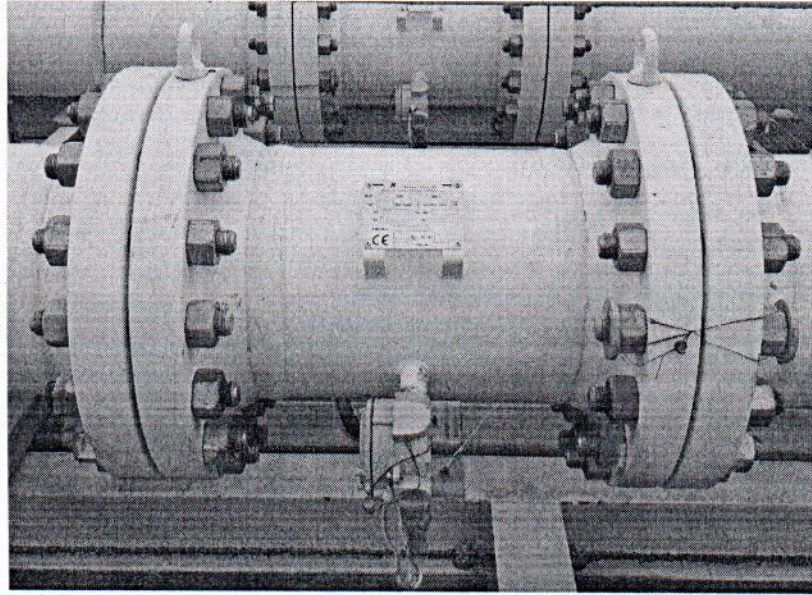
Рисунок 1.1 – Внешний вид преобразователя расхода жидкости турбинного геликоидного НТМ10 идентификационный номер Н0054
