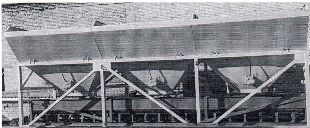
Рисунок 1.1 – Внешний вид дозатора весового дискретного действия ДВДД-И-1500 № 2103
