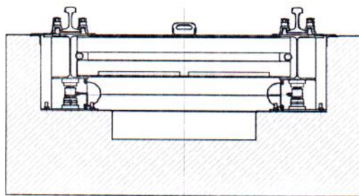
Рисунок 1 – Весовая платформа весов в поперечном разрезе.
