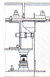
Рисунок 2 – Регулируемые винтовые упоры весовой платформы
