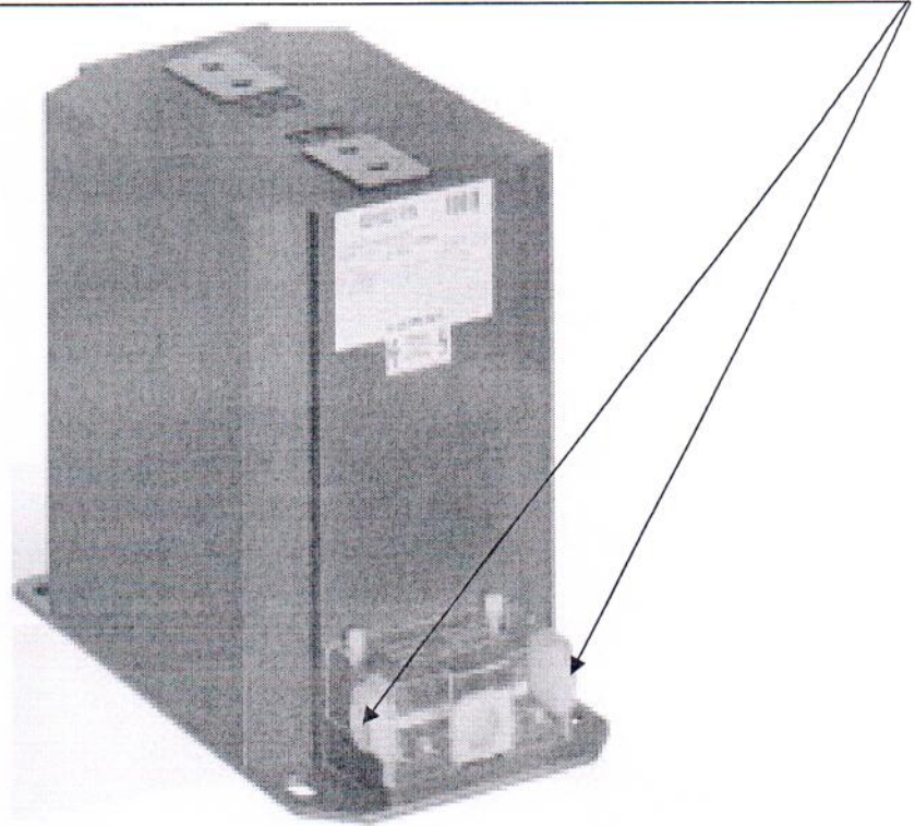
Рисунок 3.1 – Схема пломбировки от несанкционированного доступа
