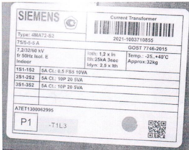
Рисунок 1.2 – Фотография маркировки трансформатора тока 4MA72-S2 АУС № 1003710855
