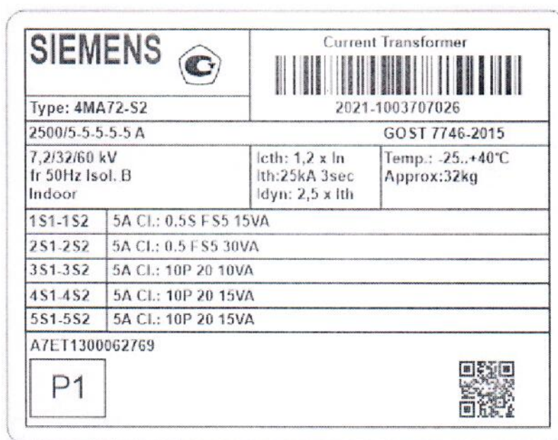
Рисунок 1.2 – Фотография маркировки трансформатора тока 4MA72-S2 АУС № 1003707026
