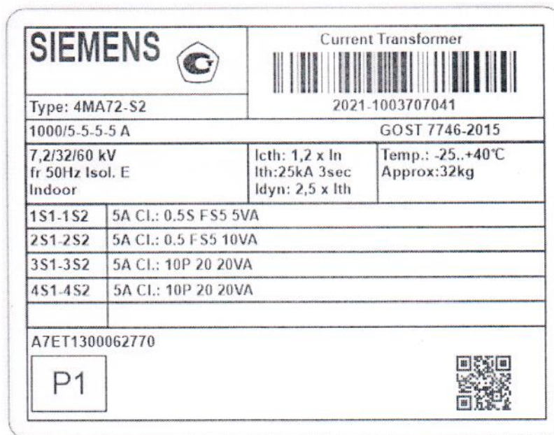
Рисунок 1.2 – Фотография маркировки трансформатора тока 4MA72-S2 АУС № 1003707041
