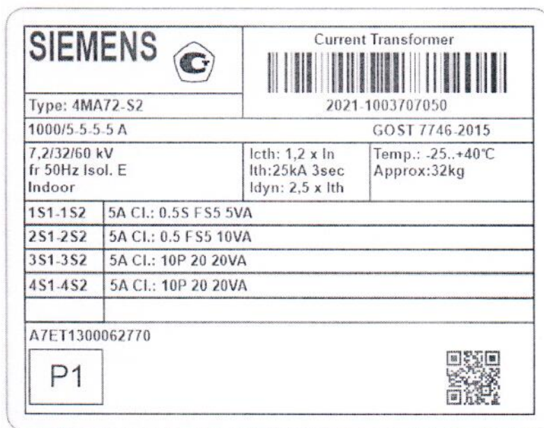
Рисунок 1.2 – Фотография маркировки трансформатора тока 4MA72-S2 АУС № 1003707050
