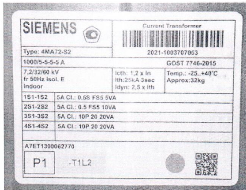
Рисунок 1.2 – Фотография маркировки трансформатора тока 4MA72-S2 АУС № 1003707053
