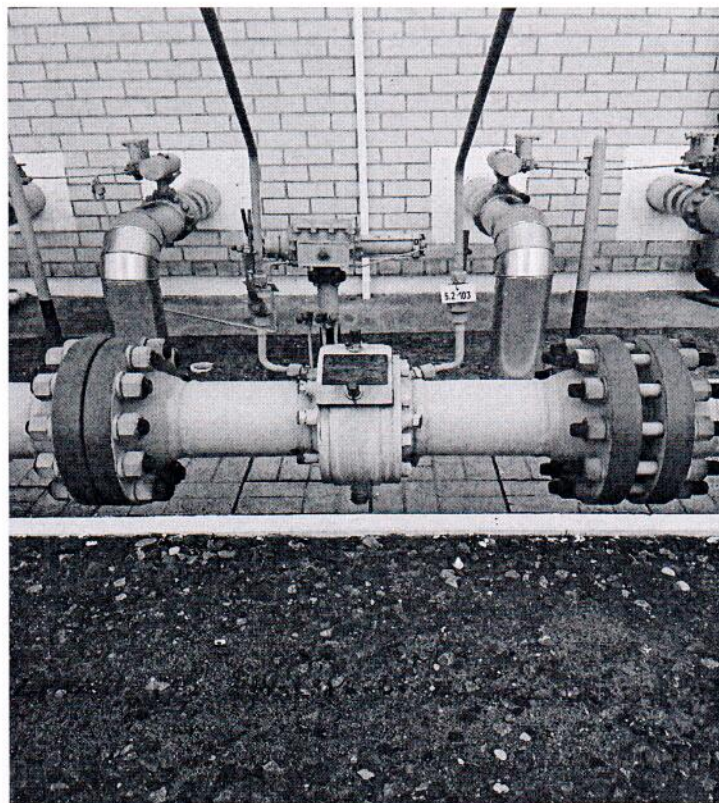
Рисунок 1.1 – Фотографии общего вида ИС УУГ
