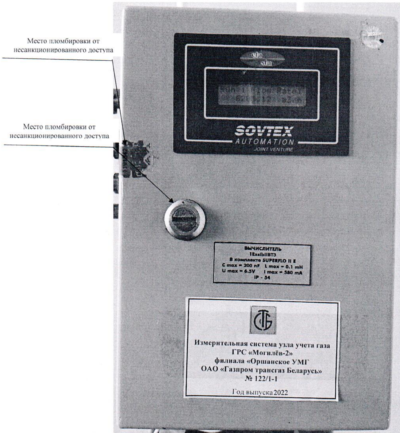
Рисунок 3.1 – Схема пломбировки от несанкционированного доступа
