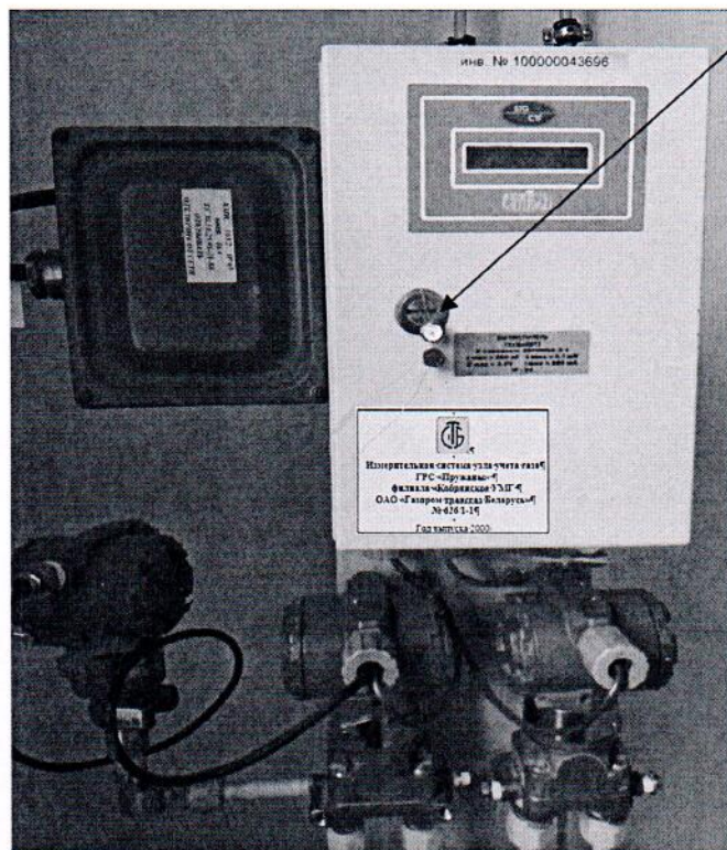
Рисунок 3.1 – Схема пломбировки от несанкционированного доступа
