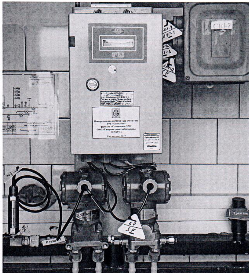
Рисунок 1.1 – Фотография общего вида ИС УУГ
