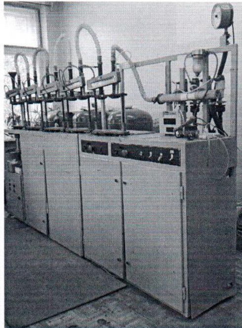
Рисунок 1.1 – Фотография общего вида стенда (изображение носит иллюстративный характер)
