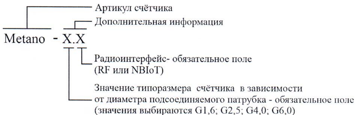
Рисунок 1 - Структура наименования и условного обозначения счетчиков
