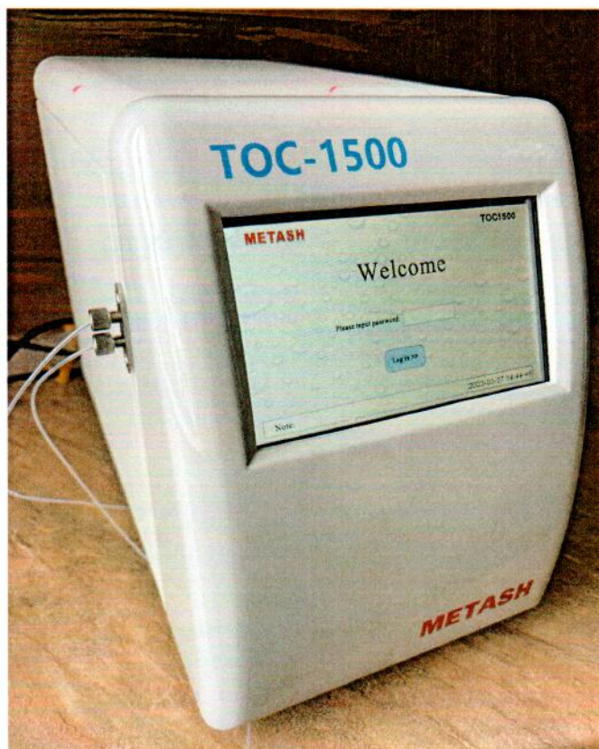
Рисунок 1.1 – Фотография общего вида анализатора общего органического углерода TOC1500 № MS-TOC-230205
