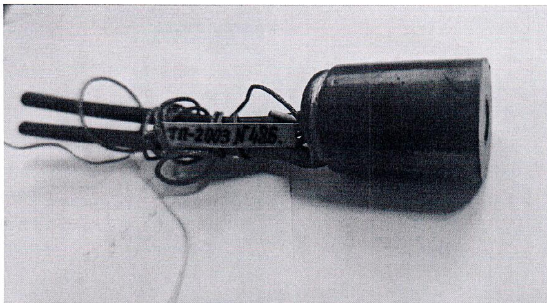
Рисунок 1.1 – Фотографии общего вида приемника теплового потока охлаждаемого ТТ-2003 № 486
