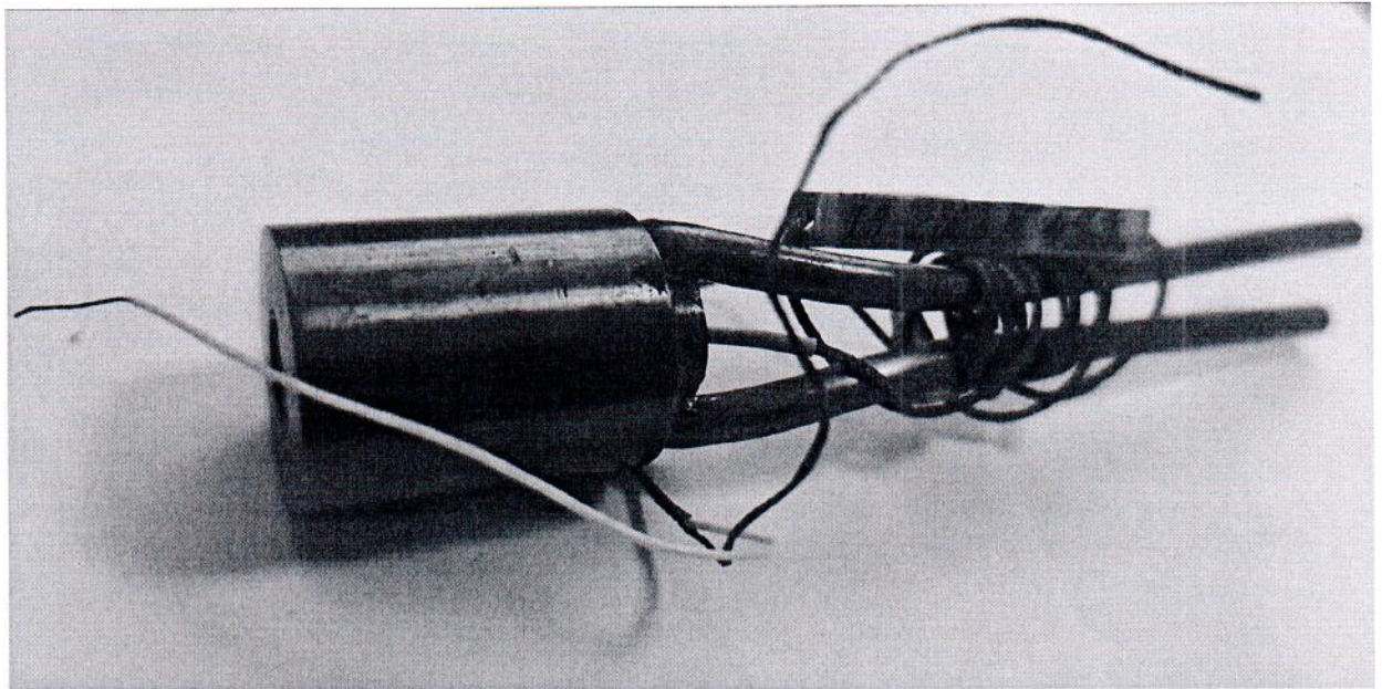
Рисунок 1.1 – Фотографии общего вида приемника теплового потока охлаждаемого ТП-2003 № 453
