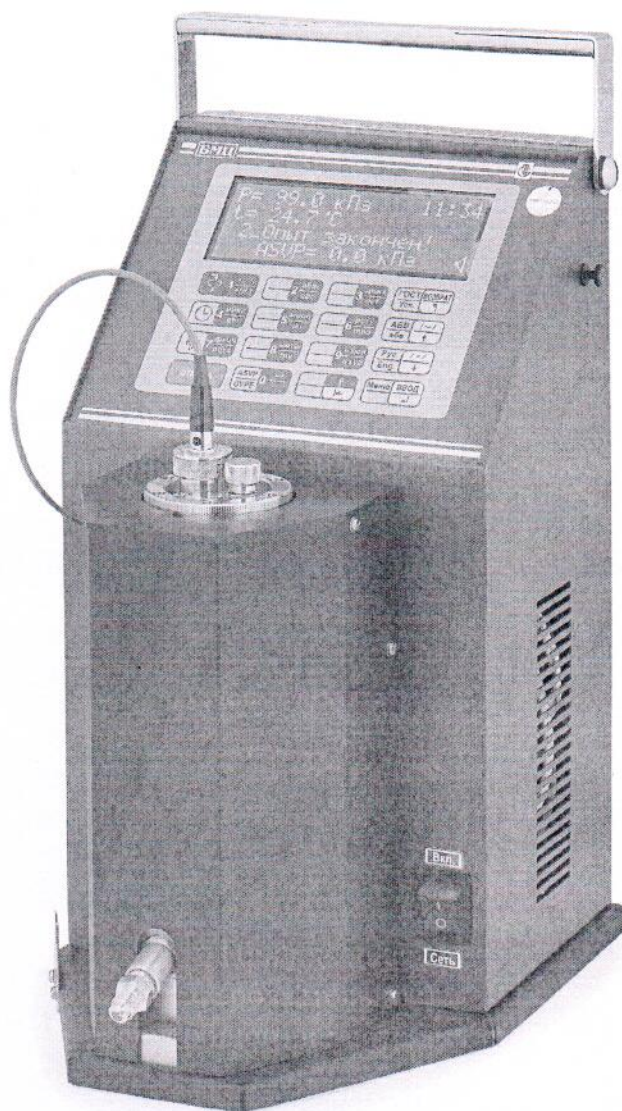
Рисунок 1.1 - Фотография общего вида анализатора давления насыщенных воздухом паров жидких нефтепродуктов АДНП
