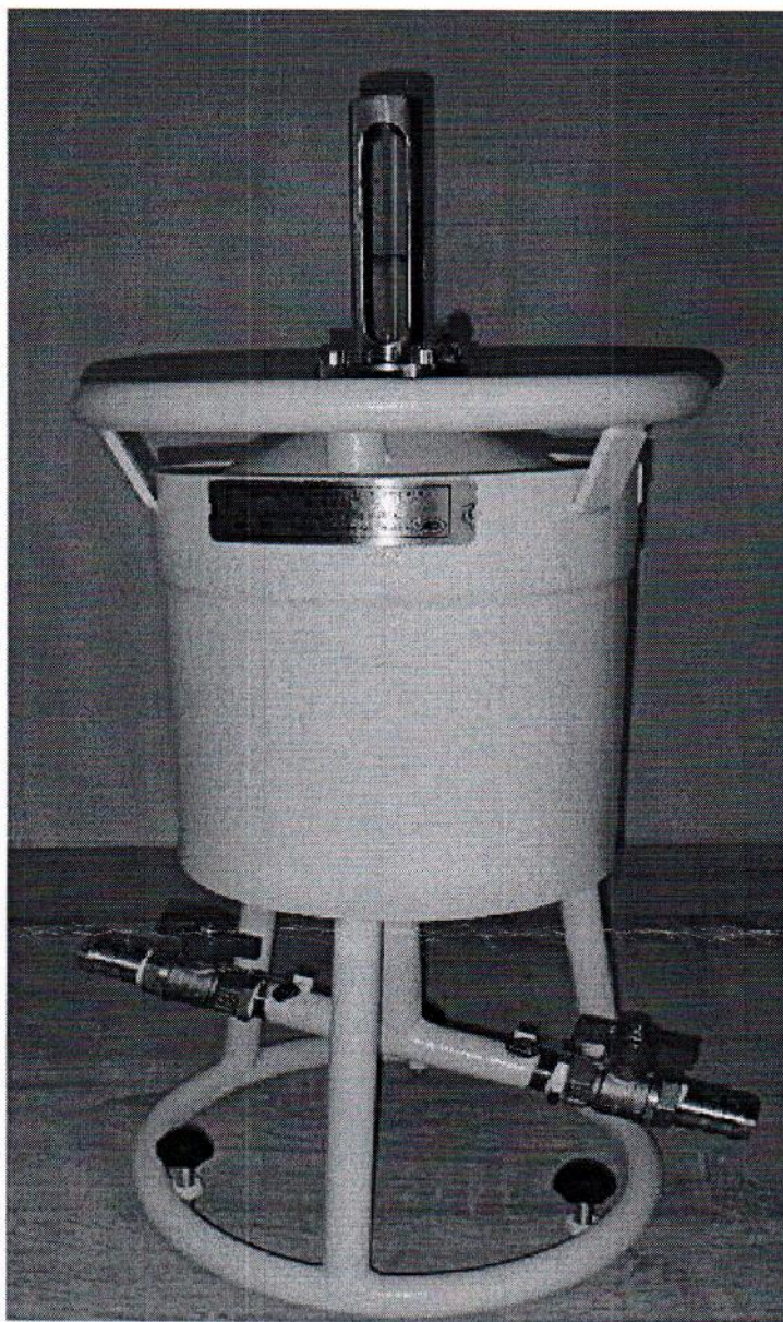
Рисунок 1.1 - Внешний вид мерника образцового 1-го разряда М1Р-5-01 № 20
