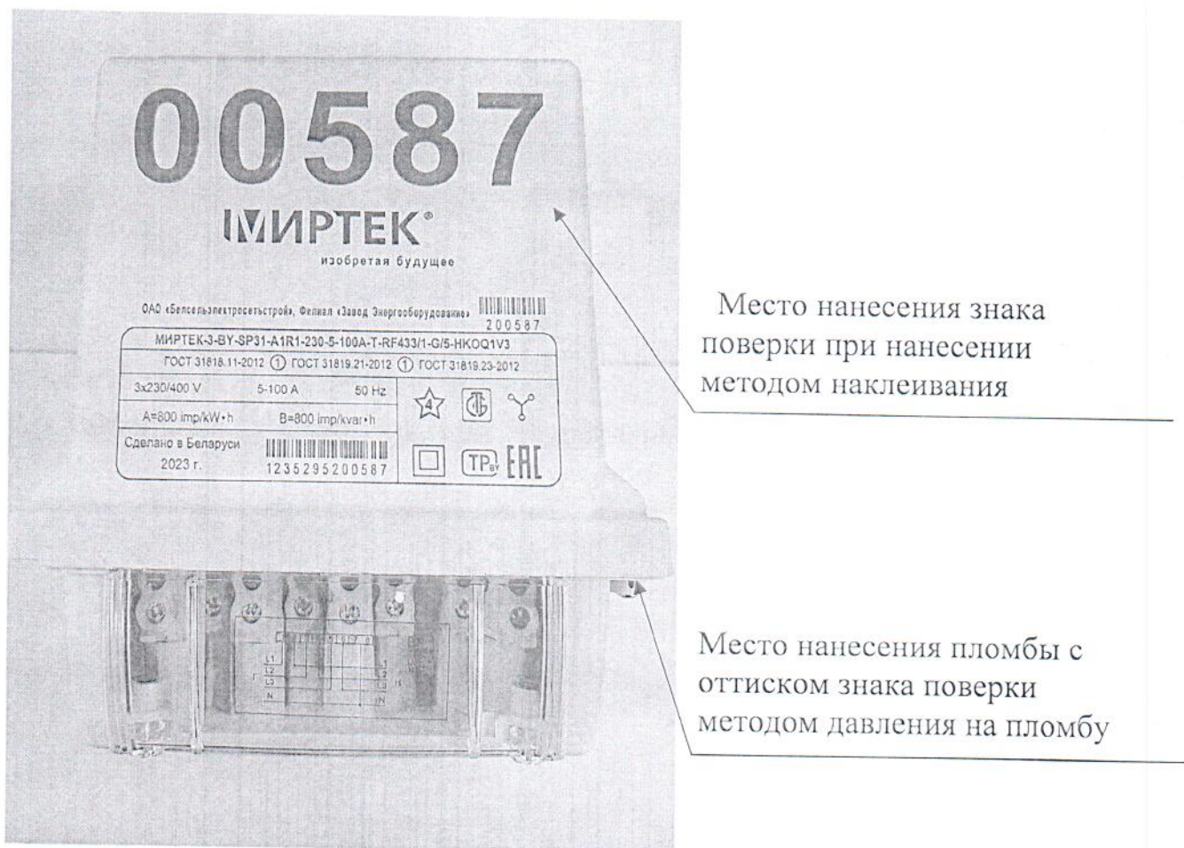
Рисунок 2.1 – Схема (рисунок) с указанием места для нанесения знаков поверки на счетчик
