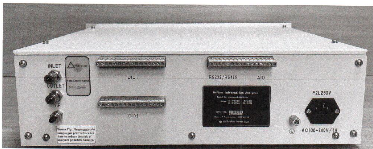
Рисунок 1.2 – Фотография общего вида. Задняя панель анализатора газа Gasboard-3000Plus, зав. № 220830140001
