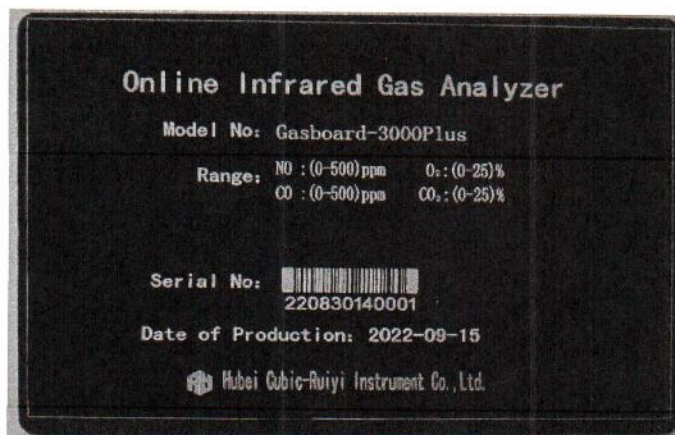
Рисунок 1.3 – Фотография маркировки. Анализатор газа Gasboard-3000Plus, зав. № 220830140001
