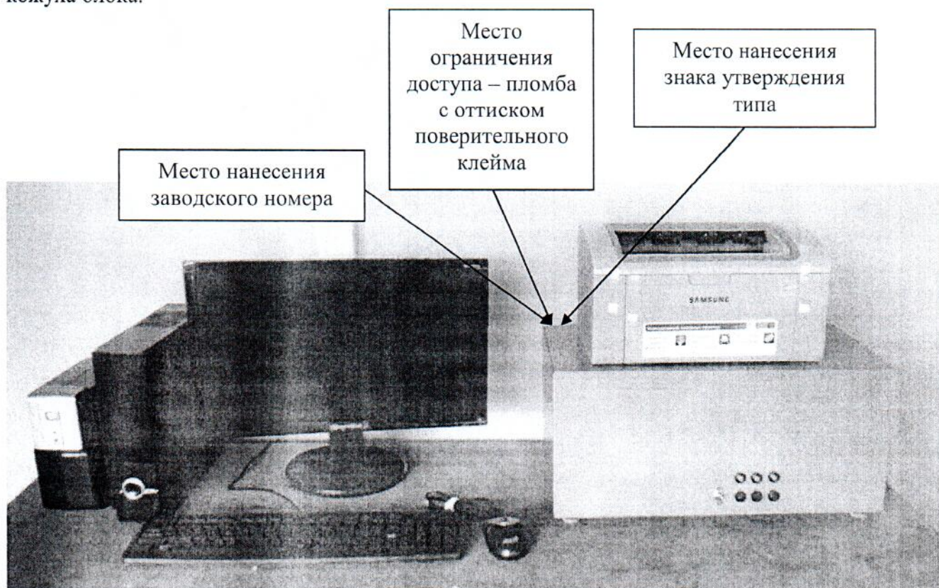
Рисунок 1 – Общий вид БЭПТ устройств УЗОТ-П с указанием места ограничения доступа к местам настройки (регулировки), места нанесения знака утверждения типа, места нанесения заводского номера
