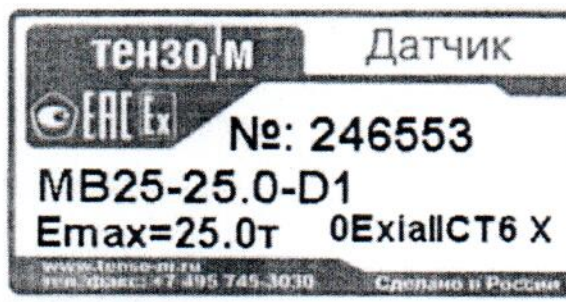
Рисунок 2 – Внешний вид наклейки датчиков
