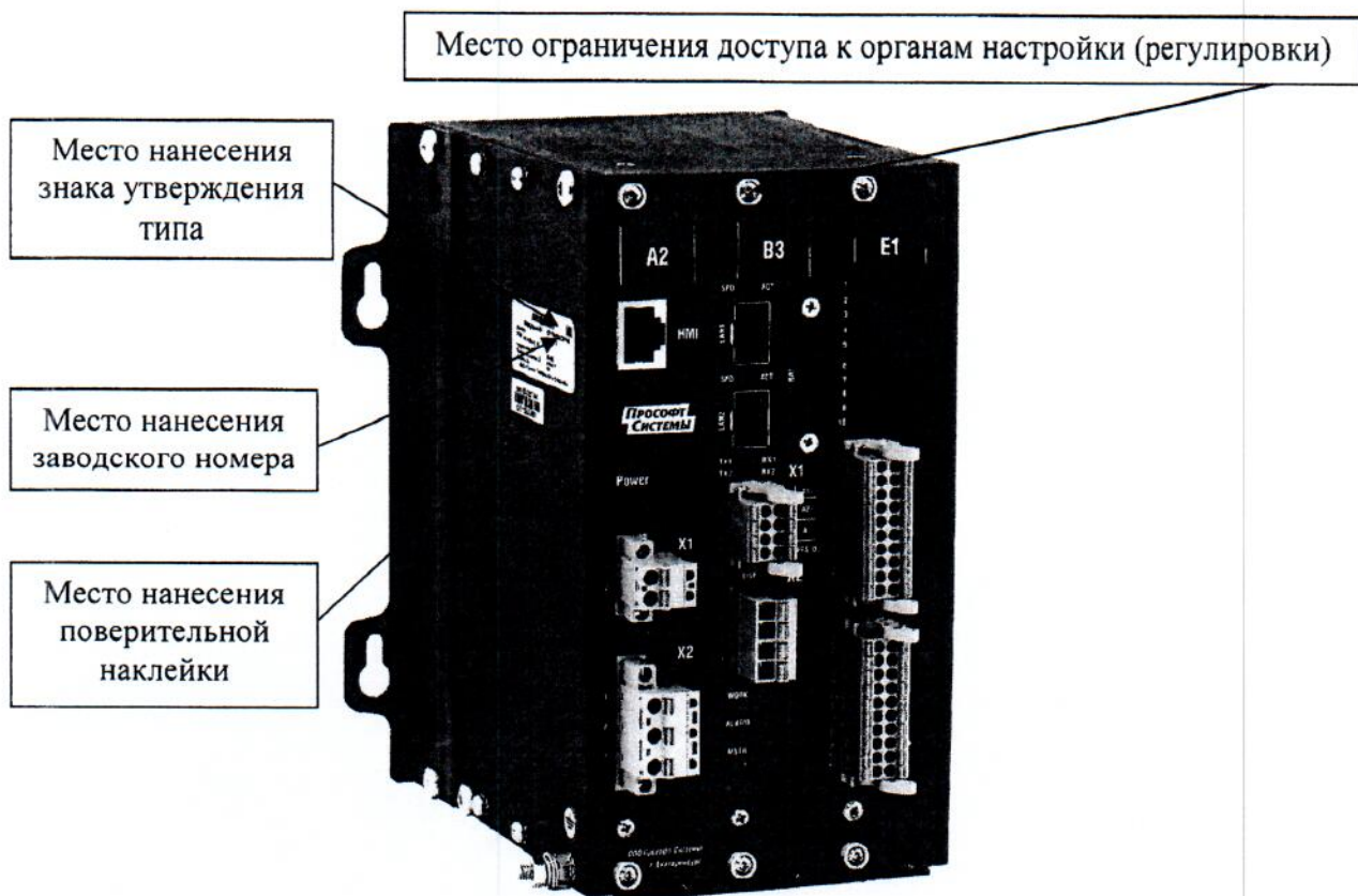
Рисунок 3 – Общий вид контроллеров исполнения ARIS-2803 (вид сзади)
