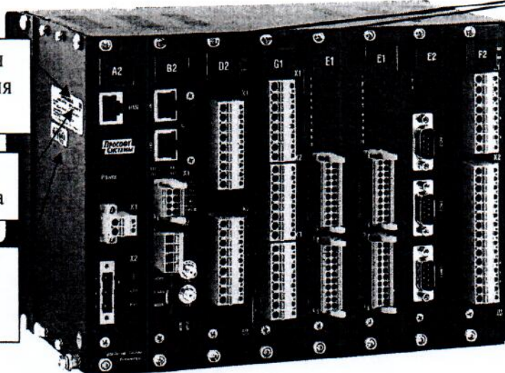
Рисунок 5 – Общий вид контроллеров исполнения ARIS-2808 (вид сзади)
