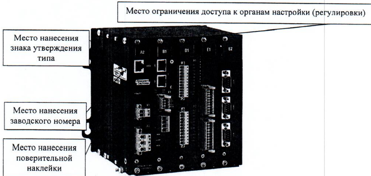
Рисунок 4 – Общий вид контроллеров исполнения ARIS-2805 (вид сзади)
