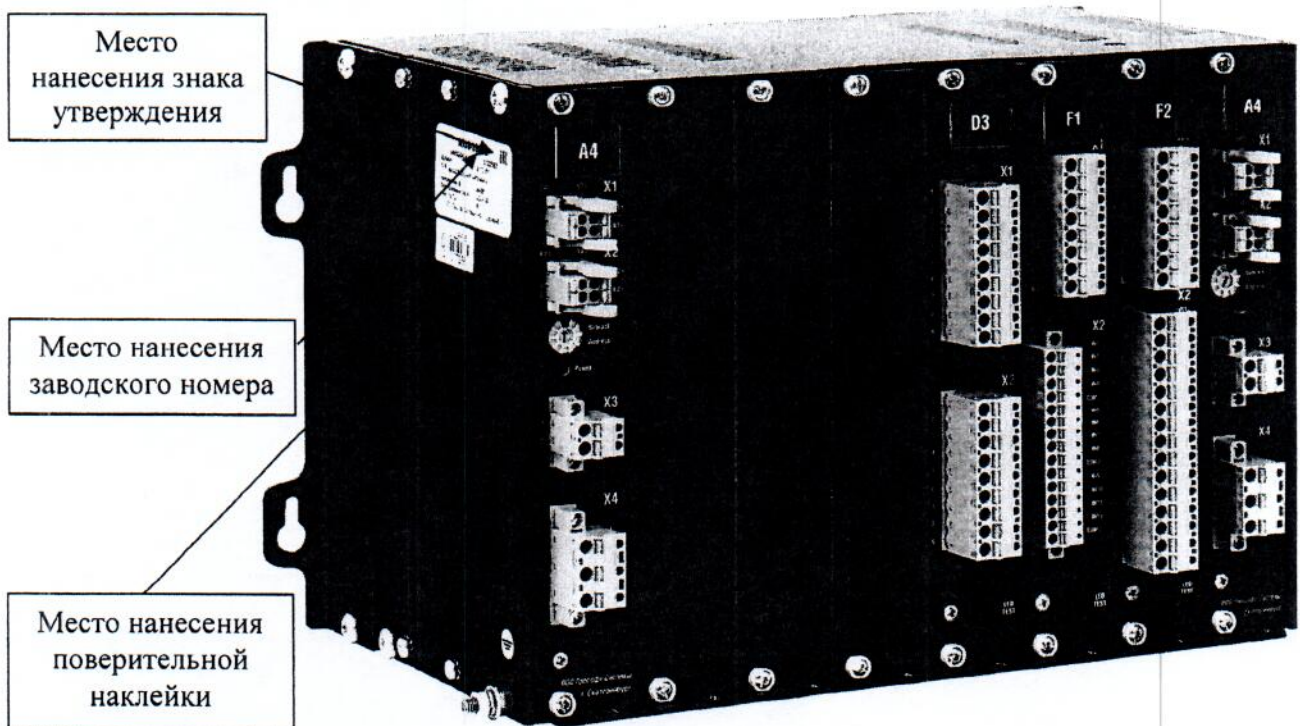
Рисунок 8 – Общий вид крейтов расширения ARIS-2808E (вид сзади)
