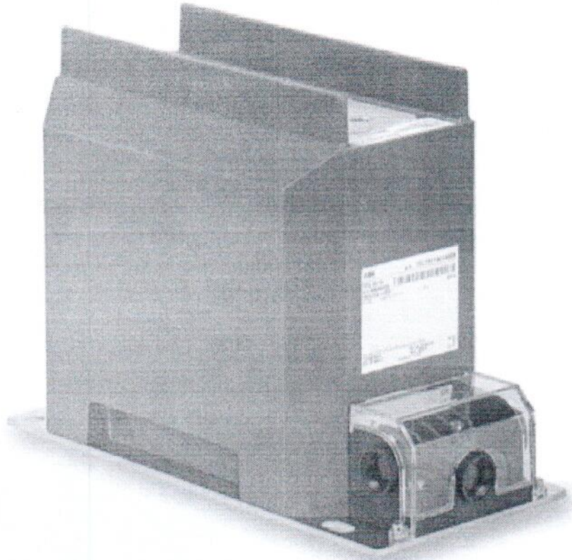
Рисунок 1.1 – Фотография общего вида трансформатора тока TRU 40.23 № 1VLT5122037547
