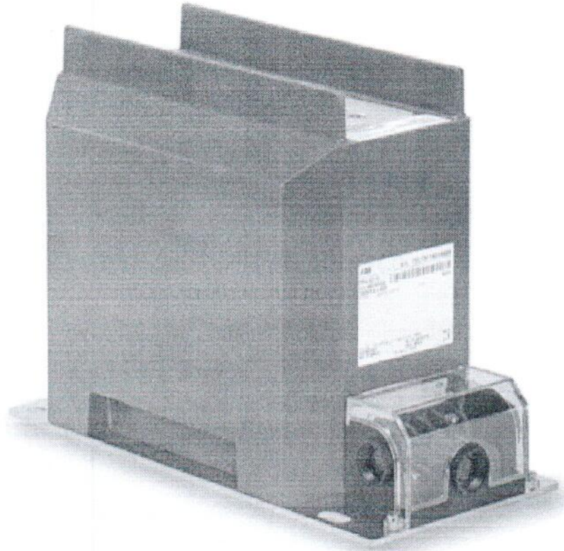
Рисунок 1.1 – Фотография общего вида трансформатора тока TPU 40.23 № 1VLT5122037541
