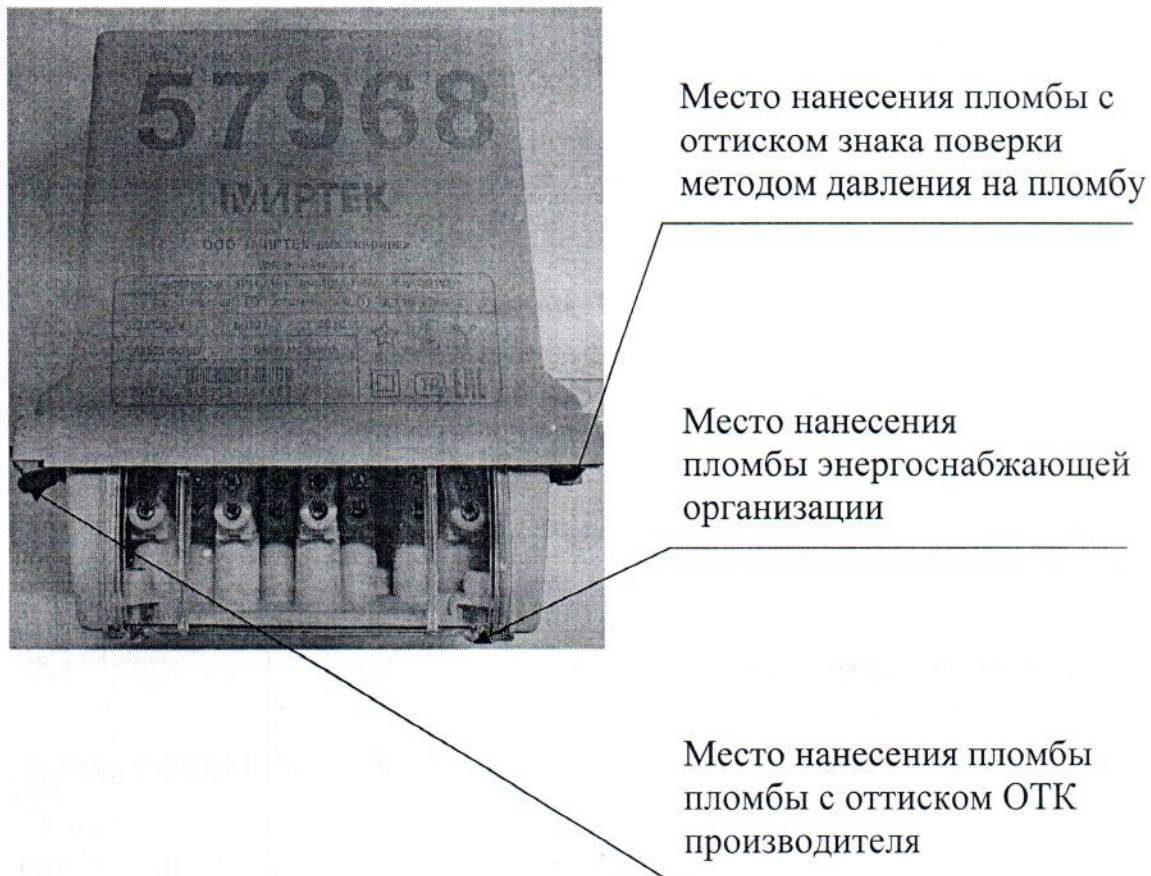
Рисунок 3.1 – Схема пломбировки счетчика от несанкционированного доступа
