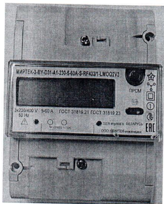
Рисунок 1.5 – Фотография общего вида счётчика в исполнении корпуса «D31» и «D34»
