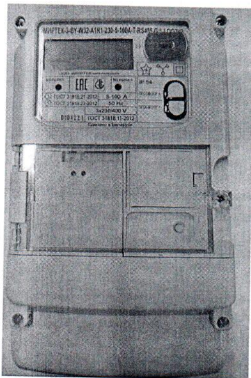
Рисунок 1.3 – Фотография общего вида счётчика в исполнении корпуса «W32», «W33», «W37», «W38»
