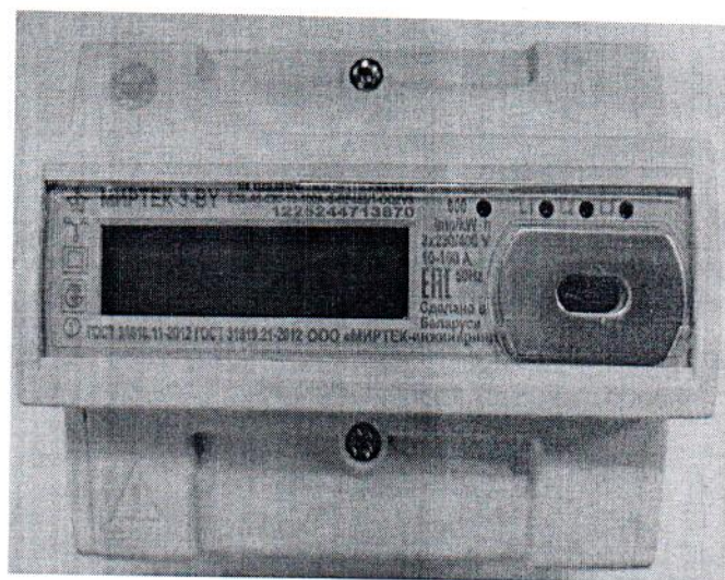
Рисунок 1.6 – Фотография общего вида счётчика в исполнении корпуса «D32» и «D33»
