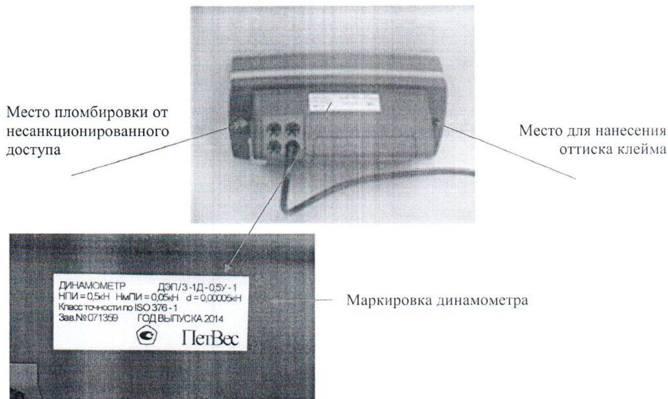
Рисунок 9. Схема пломбировки от несанкционированного доступа и обозначение места для нанесения оттиска клейма
